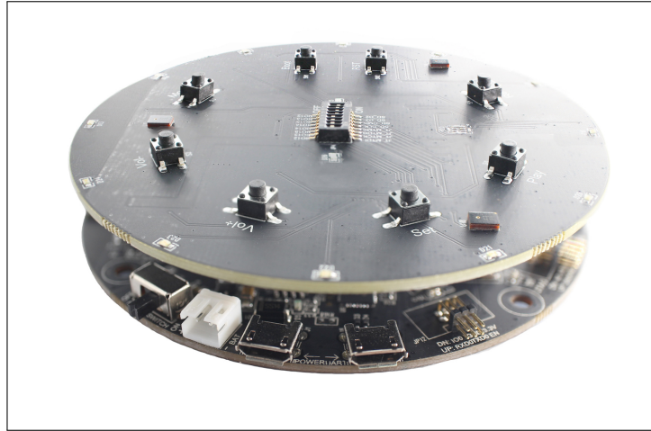
Figure 26: ESP32-LyraTD-MSC
