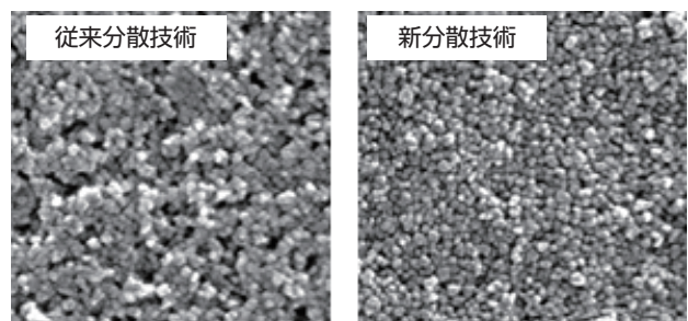
図9 テープ表面のSEM像
