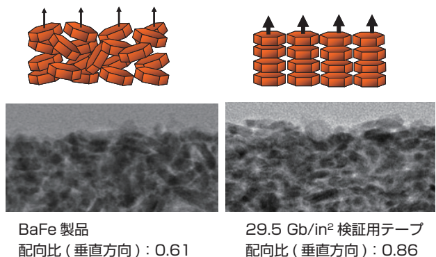
図 14 磁性層の断面の TEM イメージ [21]
